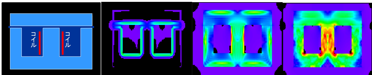
図 2 空隙のあるコアモデルと磁束密度分布の時間変化
