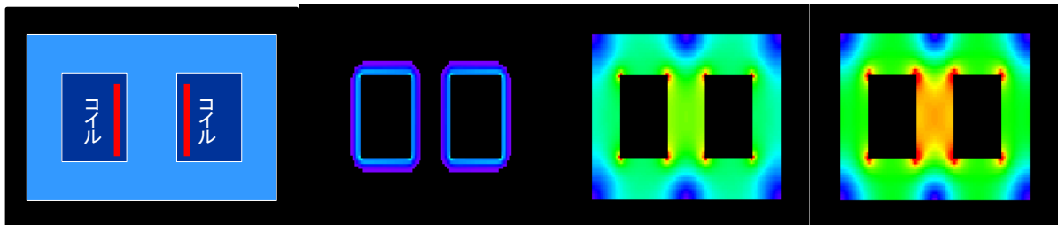
図 1 空隙のないコアモデルと磁束密度分布の時間変化
