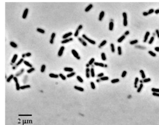
図2 n-アルカン分解硫酸還元菌 PL12 株
