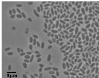
図1 トルエン分解硫酸還元菌 28bB2T 株
