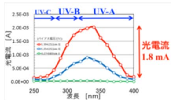
図1 ガリウム添加酸化亜鉛膜の光スペクトル
