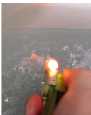
写真 1 水面にライターで着火した様子
