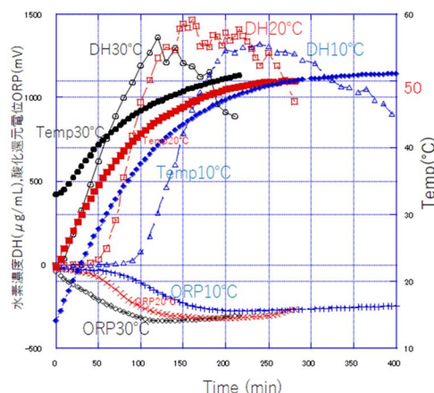
図 1 初期水温の違いによる溶存水素濃度 (DH)、酸化還元電位 (ORP)、水素の経時変化
