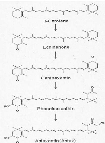
図2 アスタキサンチンの合成経路
