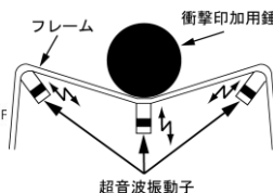
図-3 衝撃吸収装置
