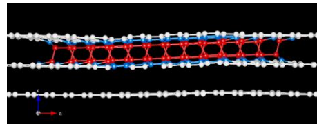
図1: グラファイト中に光誘起されたダイヤモンドドライドメイン (Diaphite)の構造(数値計算結果)
