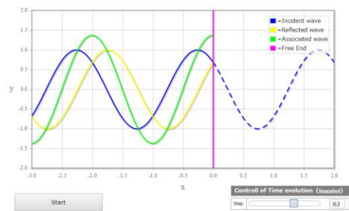
図 4: 正弦波の自由端反射
