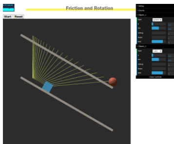
図 2: 斜面上の物体
