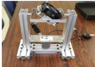
図2 小型軸流ファンの振動計測
