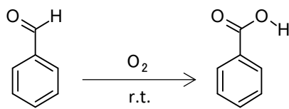
図 1 ベンズアルデヒドの酸化反応
