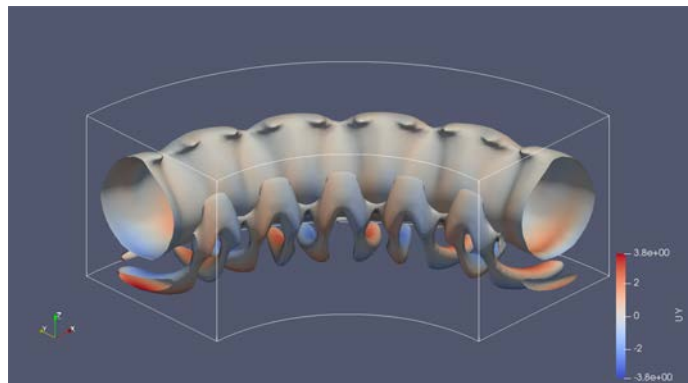
図 2 対流構造
