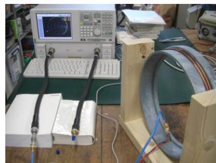
図1 実験環境
