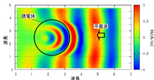
図3 FDTD 法による計算例
