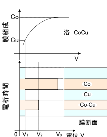
図1 電析法による多層薄膜作製
