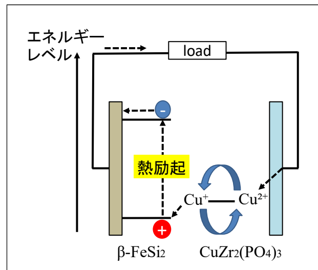
\beta\text{-FeSi}_2/\text{CuZr}_2(\text{PO}_4)_3 層状増感型熱発電素子の発電原理
