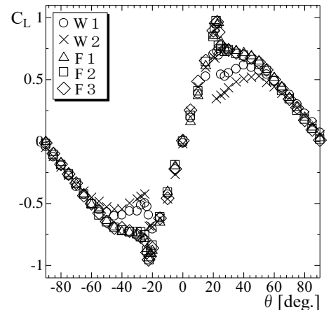
図. Lift Coefficient の例
