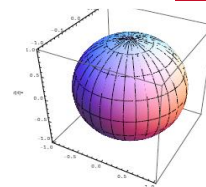
対称空間の例 2次元球面
