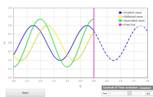
図3: 正弦波の自由端反射
