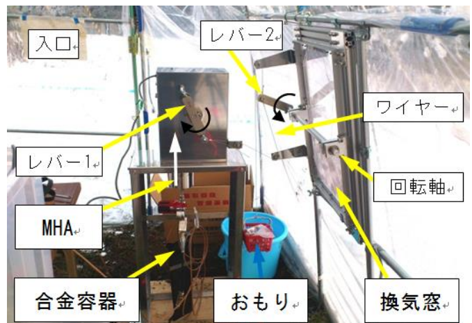
図3 MHA 駆動型ビニールハウス用窓開閉装置
