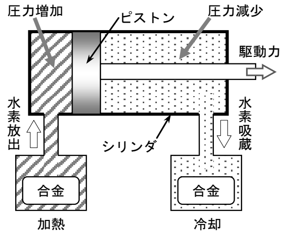
図1 MHA 概略図
