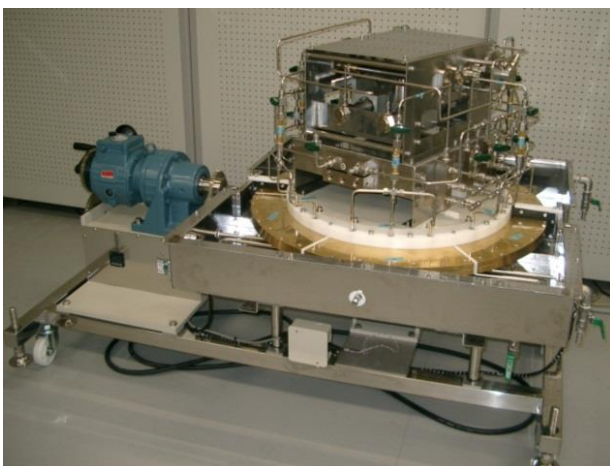
図2 自立駆動型 MHA の試作機
